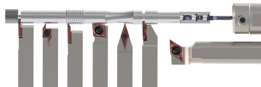
▶ Dụng cụ cắt cho máy tiện tự động Cutting tools for automatic lathes
