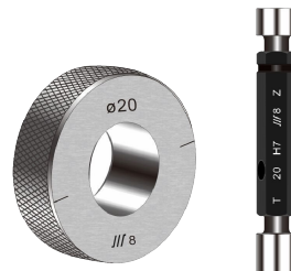
▶ Dưỡng kiểm trục/lỗ Pin gauge
